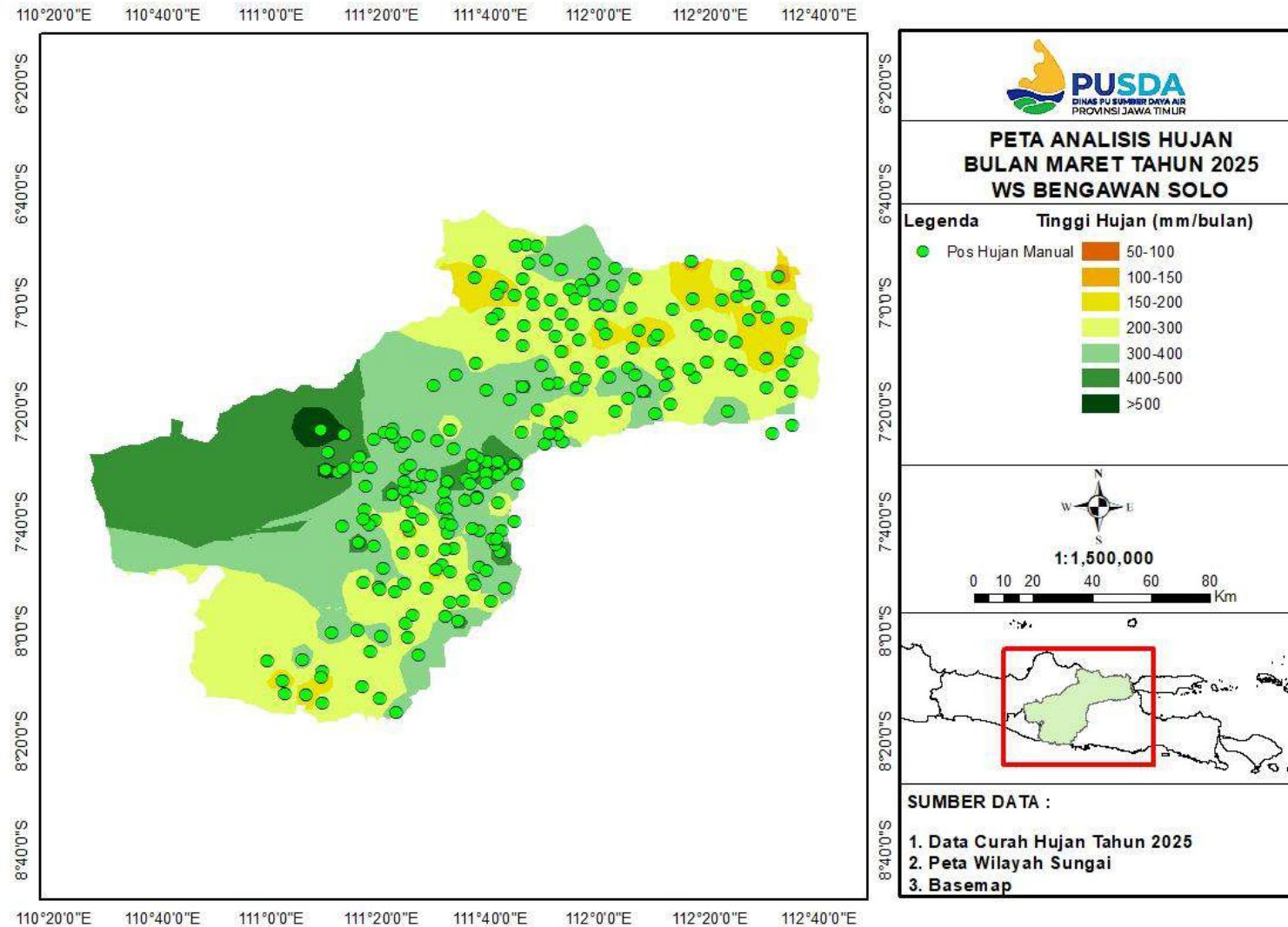
Gambar 4.4 Peta Analisis Hujan Bulan Maret Tahun 2025 WS Bengawan Solo
